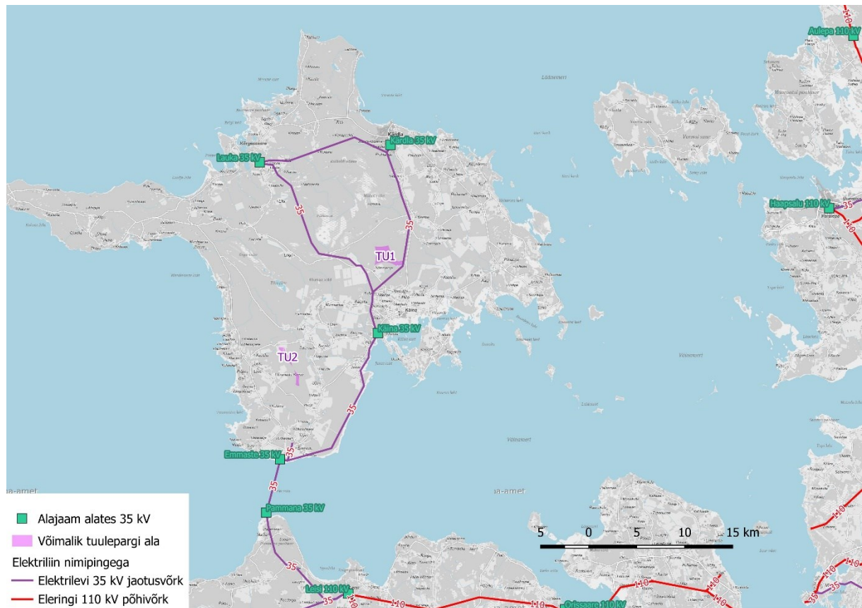
Joonis 11. Hiiumaa elektrihüvendust tagav liinivõrk ja uuringu I etapi analüüsis selgunud tuulepargi arendamiseks sobilikud alad.
