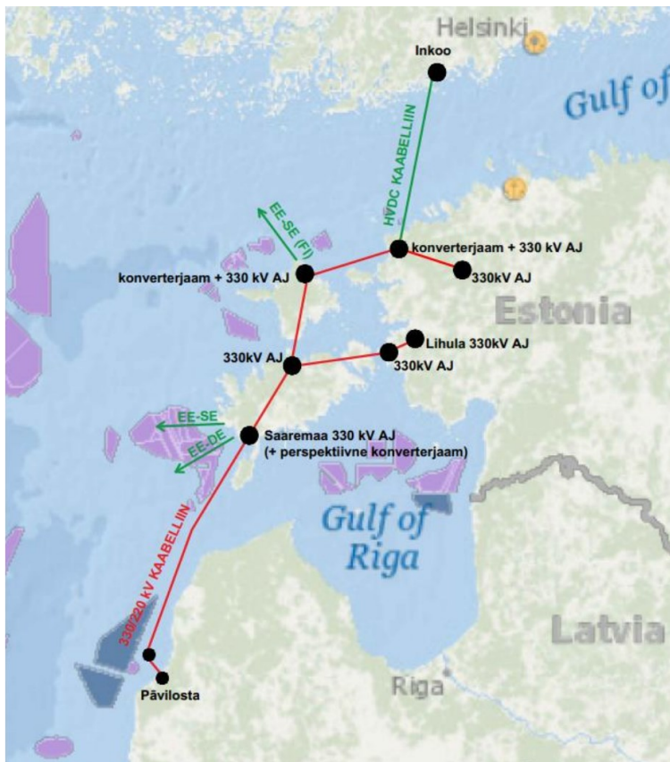
Joonis 16. Võrgu pikaajaline tulekuvision (Eesti elektriülekandevõrgu arengukava 2024-2033).
