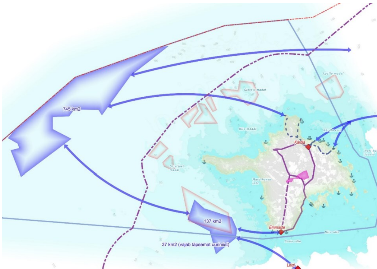
Joonis 17. Potentsiaalsed meretuuleparkide arendusalaad (sinisega) ja kaabelühendused (sinised nooled). Punaka tooniga on märgitud uuringu koostamise ajaks esitatud tuuleparkide hoonestuslubade taotlused. Ruumiline eelanalüüs Hiiu merealal tuuleenergeetika alade planeerimiseks 2022.
