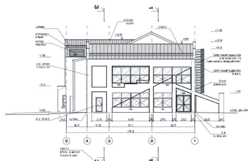
▼ LÄÄNEFAASID (L) ja varisnõu (V) koos varisnõu ehk vaade tänava poole
