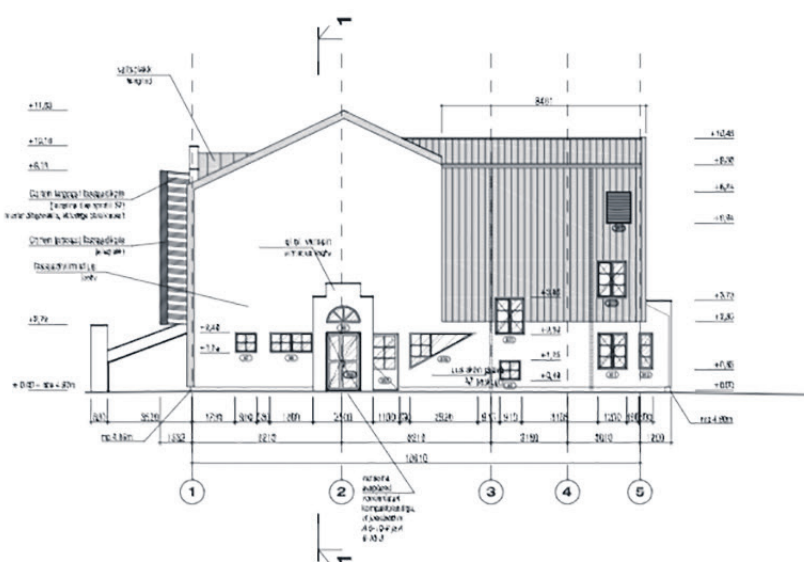
▼ IDAFaasid (I) ja varisnõu (V) ehk vaade garaaži poole
