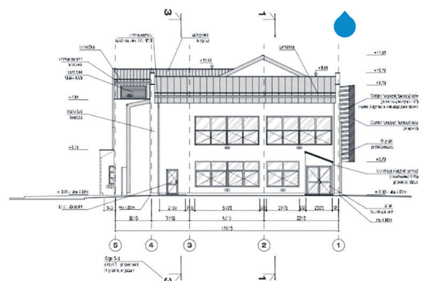
▲ LÄÄNEFAASID (L) ja varisnõu (V)
